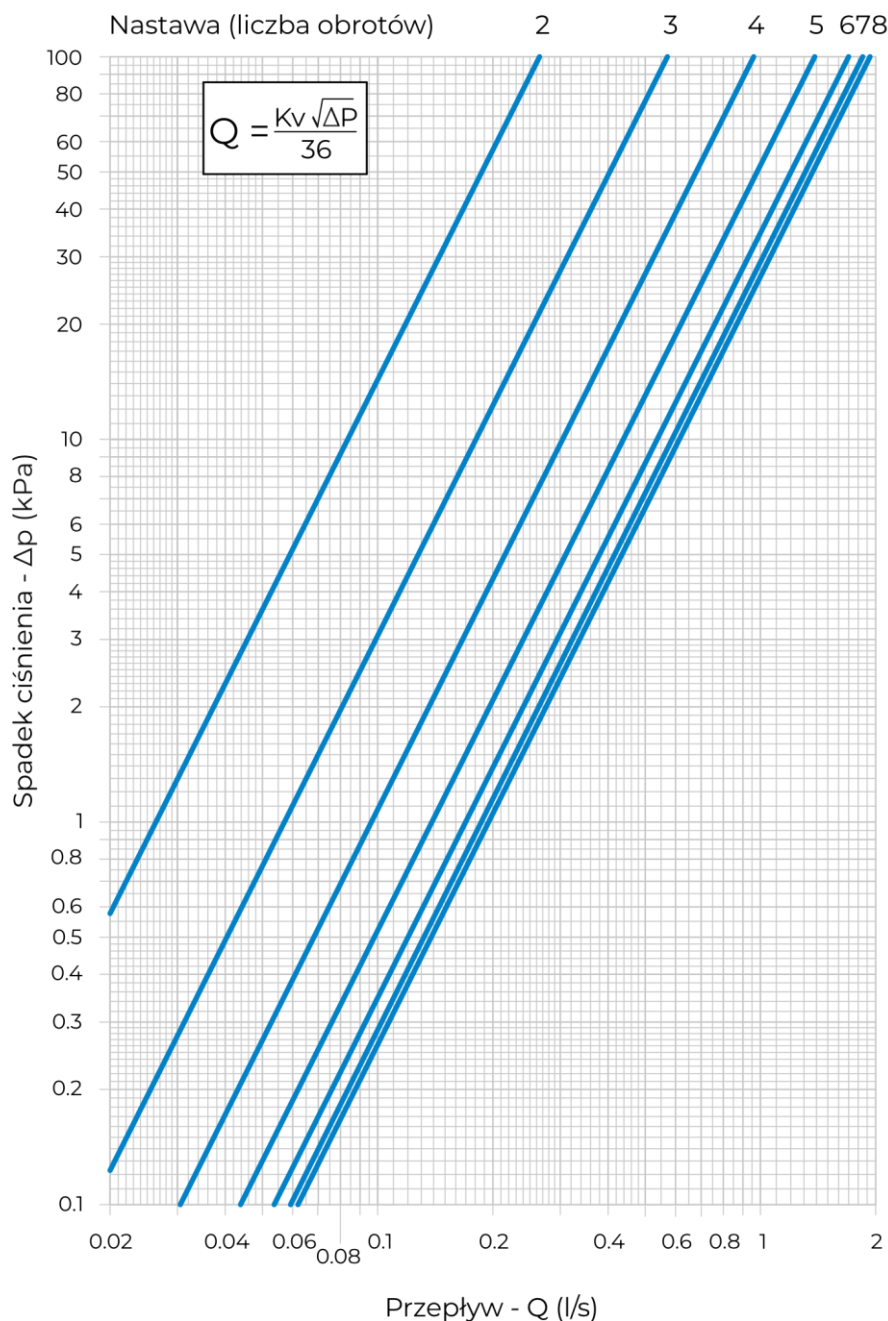
Kv (przepływ w m³/h przy spadku ciśnienia 1 bar)
