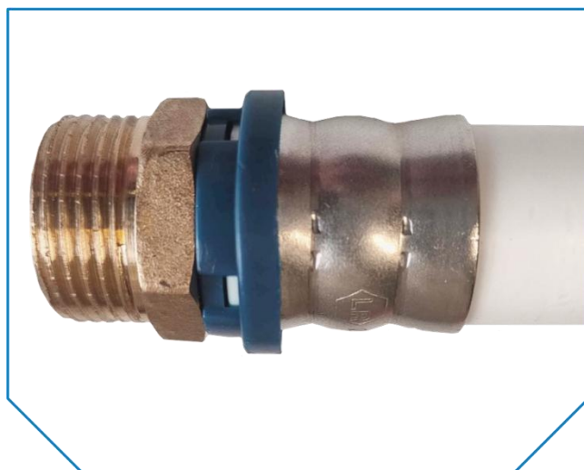
Przyłożenie szczęki „U” do złączki na rurze o średnicy 25 mm. Widok 2 w zaciskarce.
